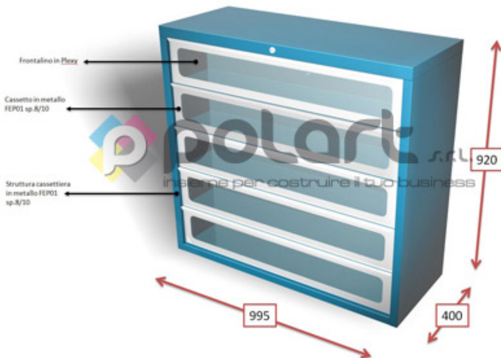
Rendering Cassettiera in metallo
